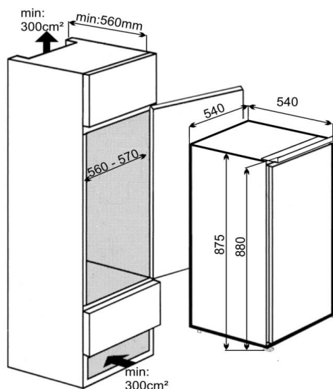
EKS 145-11 A+
