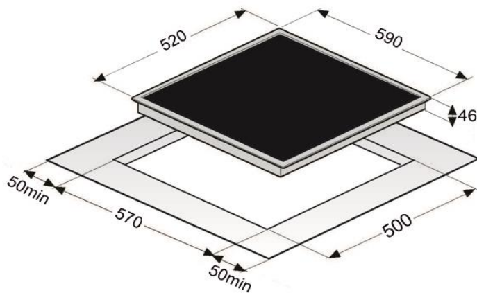
Einbauskizze
