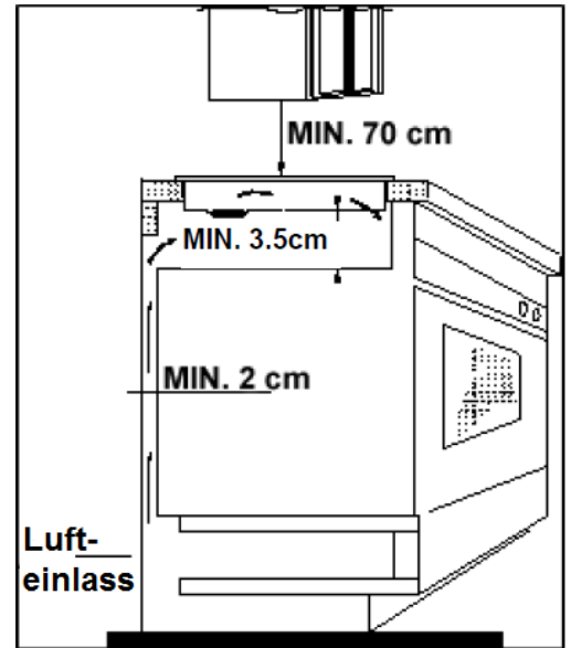
Abbildung 1 Einbau
