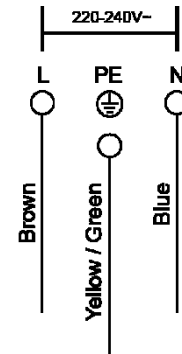
Abbildung 4 Anschluss N1
