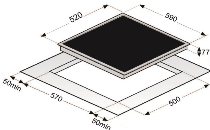
Einbauskeizze
