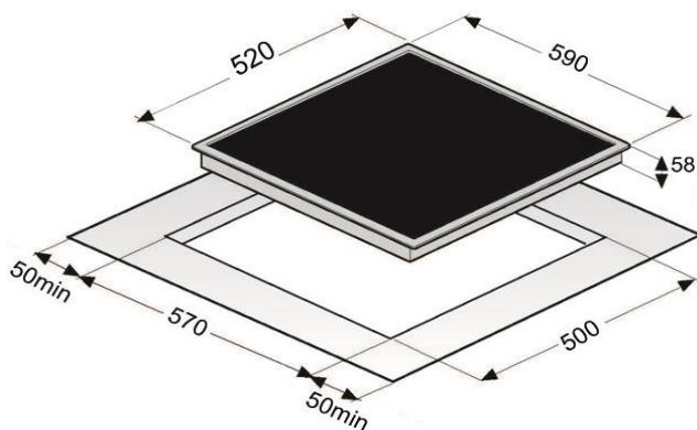
Einbauskeizze
