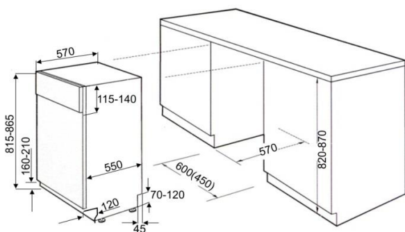
Einbauskizze
