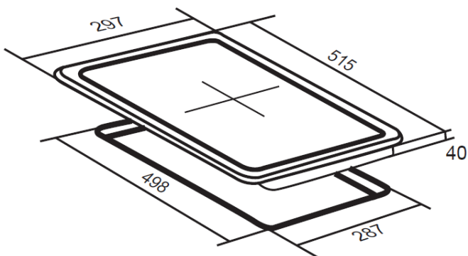
Einbauskizze
